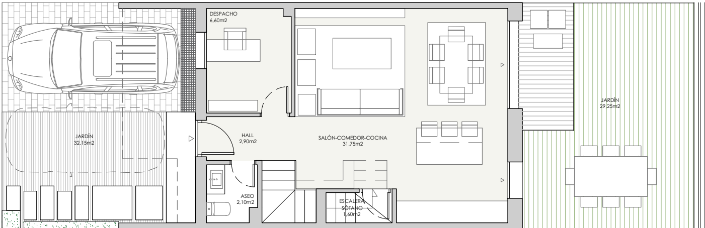
PLANTA BAJA
